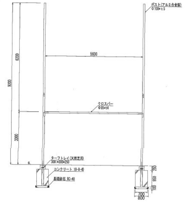
ラグビーポスト詳細図
